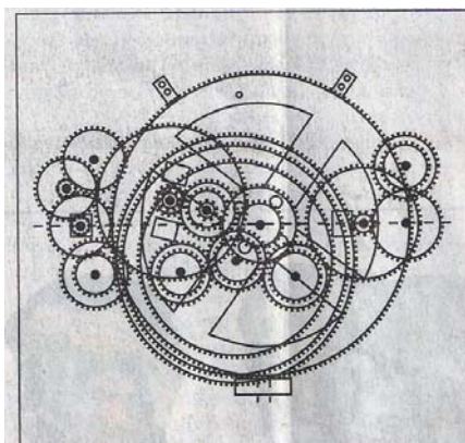
Das Innenleben des Sternrechners: Fast 40 ZAHNRÄDER griffen ineinander
