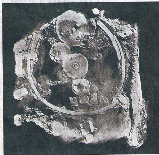
Feine Zacken unter Grünspan und Patina: Das RÖNTGENGERÄT macht sie sichtbar
